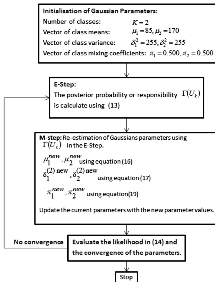
Figure 4 The EM algorithm summary. The steps of EM algorithm.
